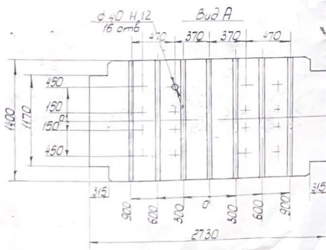
Рис 25 Эскиз межпанельного пространства
