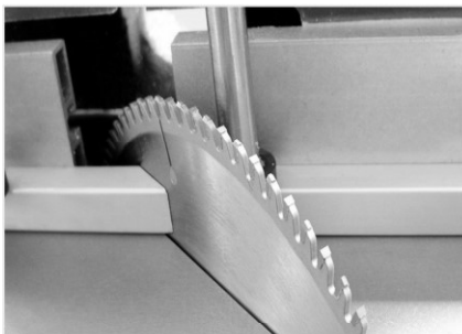
Sega a tavolo TS 161/21
