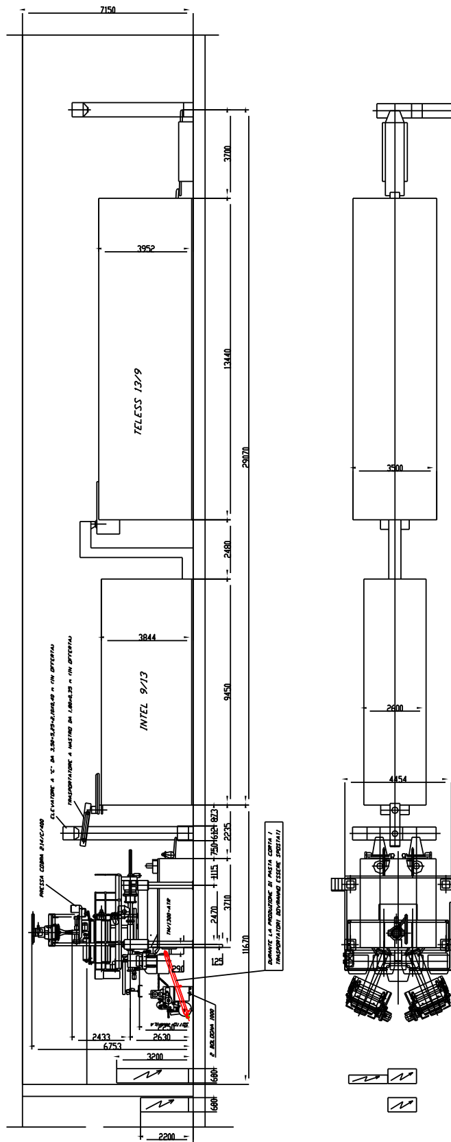
PDS. 5 LINEA AUTOMATICA CONTINUA PRODUZIONE PASTA CORTEA composta da:
