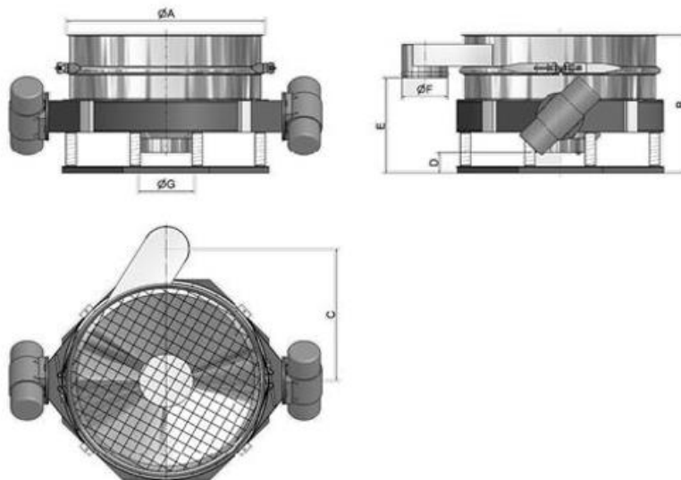
Abbildung 3Körper Rundrüttlersieb Serie MSC
