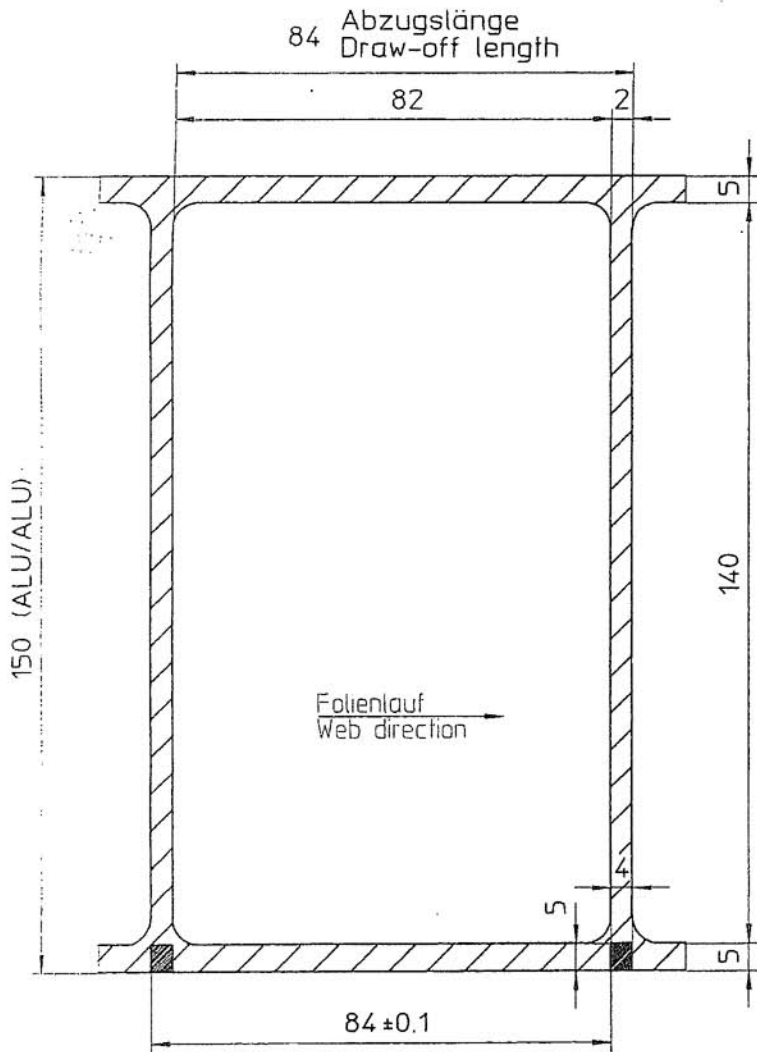
Ansicht auf Deckfolienseite. View on lidding foil.
