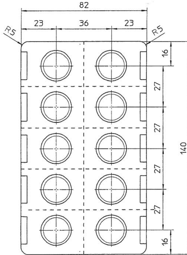
Ansicht auf Deckfolienseite. View on lidding foil.
