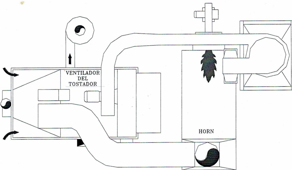
DISEÑO N° 40893
